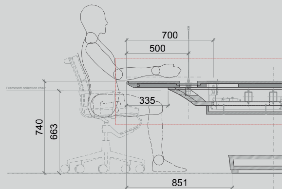
3 COUPE A-A ECHELLE 1:20
